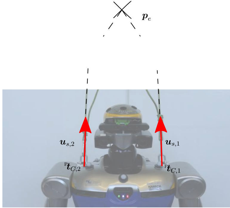
FIGURE 2.4 – Grandeurs utiles pour le modèle de contacts au niveau des épaules : \mathbf{p}_e est la position du point d’ancrage des cordes au plafond, {}^P \mathbf{t}_{C,i} avec i \in \{1, 2\} représente la position dans le repère proprioceptif des points d’ancrage des cordes au niveau des deux épaules, \mathbf{u}_{s,i} avec i \in \{1, 2\} représente les vecteurs unitaires donnant la direction des cordes dans le repère monde.
