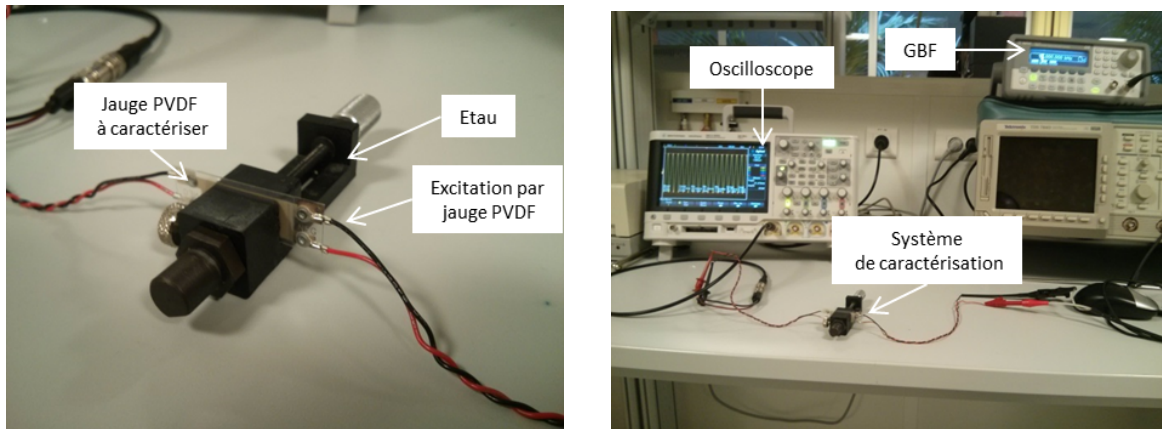
(a) Films LDT28K-01 montés sur l'étau
