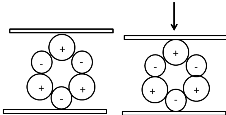
FIGURE 2.1 – Structure piézoélectrique élémentaire soumise à un effort mécanique
