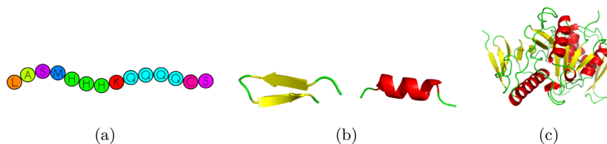
Figure F.2: Structure primaire (a), secondaire (b) et tertiaire (c) de la protéine. En (b,c), les hélices \alpha sont représentées en rouge et les feuillets \beta sont marqués en jaune.
