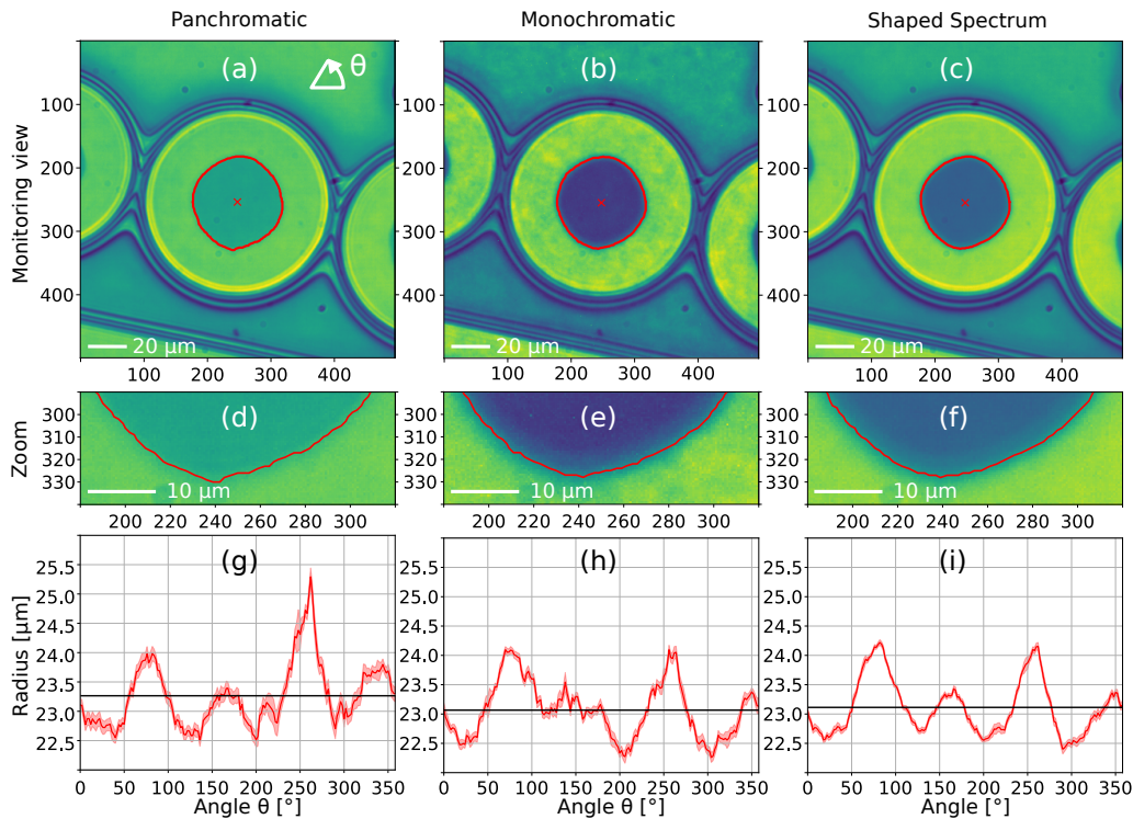
Figure 4.16: Détection du front d'oxydation pour les trois spectres d'illumination: panchromatique [(a), (d), (g)], monochromatique [(b), (e), (h)], et structuré [(c), (f), (i)]. A partir des vues [(a)-(c)] un fonction d'erreur a été fittée pour déterminer la position du front d'oxyde (ligne rouge), présentée en coordonnées polaires en [(g)-(i)]. La largeur de l'intervalle de confiance à 95% sur la détection de cette position par le fit est montrée par la zone rouge claire. Le rayon moyen détecté est représenté par la ligne noire. Figure provenant de [9].
