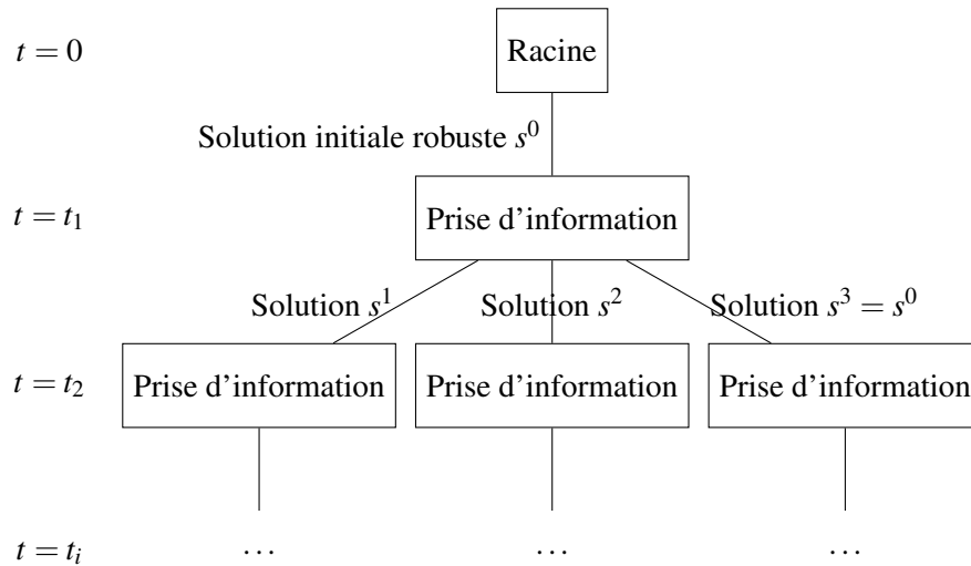
FIGURE 3.1 – Idée générale des arbres de décision robuste.
