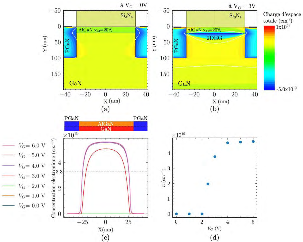
FIGURE II.21 – Simulation de la charge d'espace totale d'une cellule avec une tension V_G (a) de 0 V et (b) de 3 V ; (c) Profil de concentration du 2DEG pour plusieurs tensions V_G et (d) Évolution de la concentration moyenne \bar{n} du 2DEG en fonction de V_G
