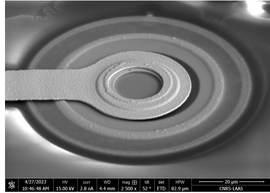
(b) Zoom on the EAM mesa.
