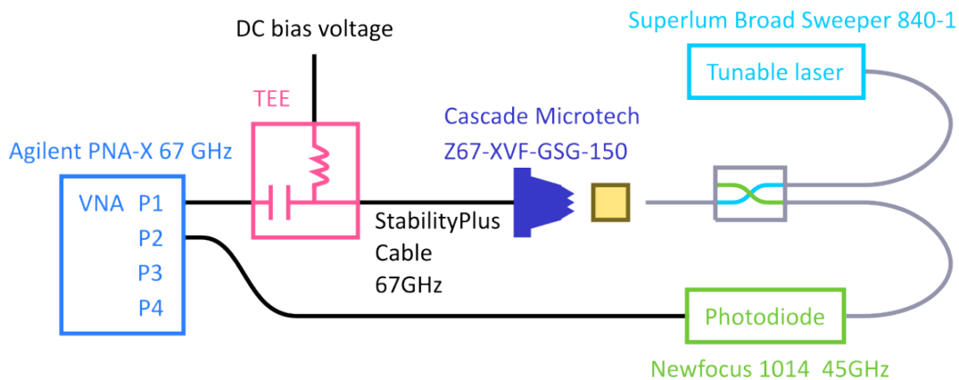
Figure 8: Schéma de la caractérisation électro-optique de l'EAM avec un VNA et une injection laser externe.
